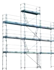
Echafaudage de façade cadre en «H»
